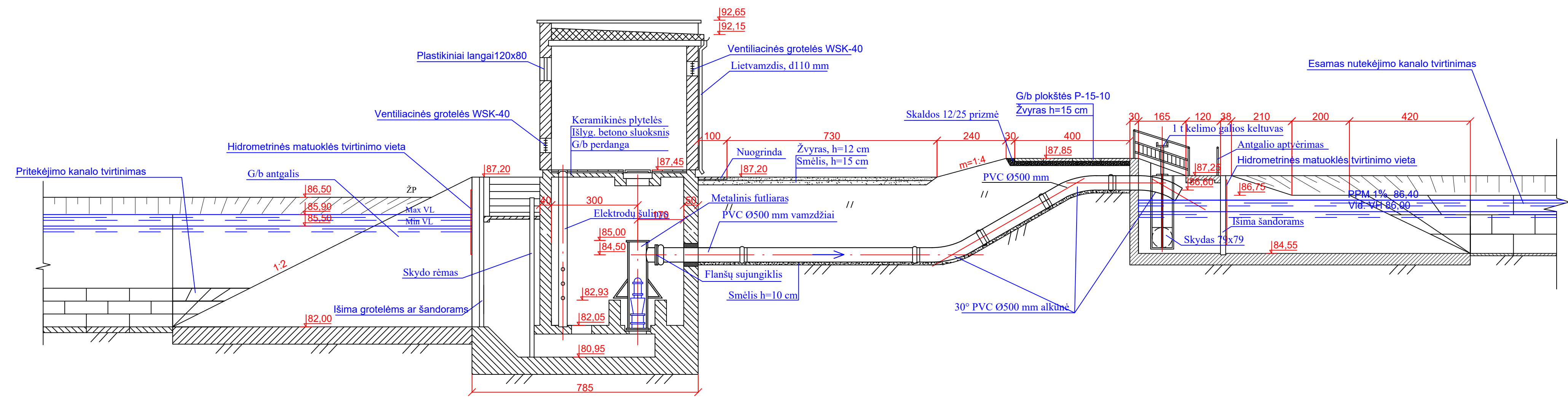
Pjūvis 1-1, M1:100
